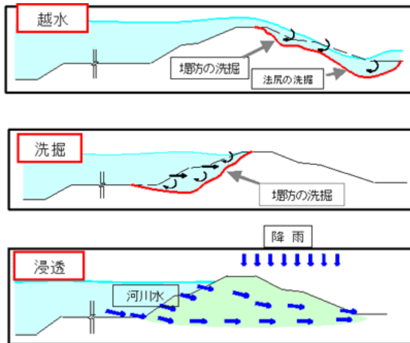
図 3-19 堤防の決壊メカニズム
